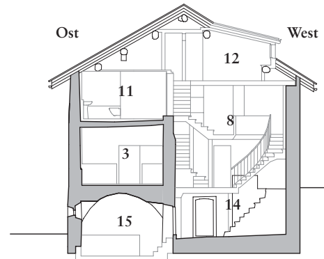
Querschnitt A
